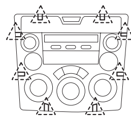
センターパネルモジュールのクリップ位置
