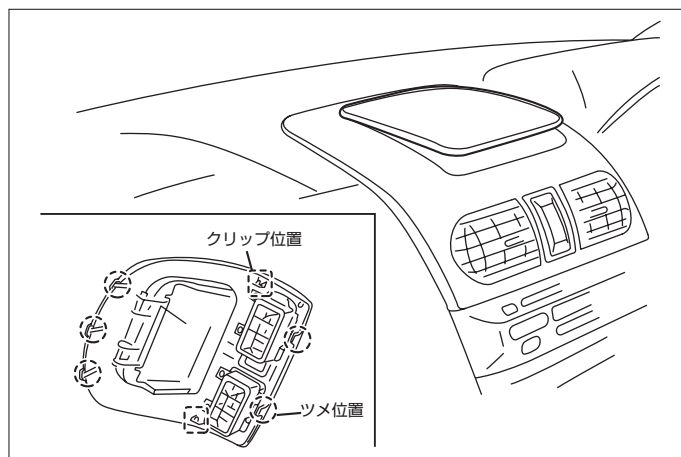
(2) クラスタリッドCを取外します。
