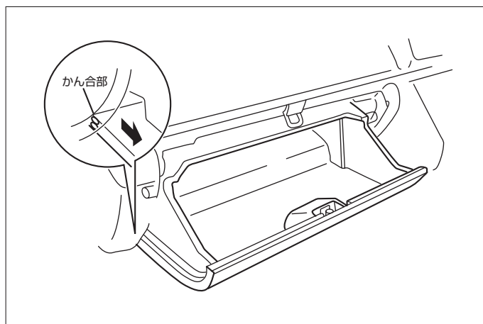
(2) グローブボックスをいっばいに下げます。
