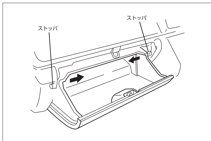
(1) グローブボックスを開け、ストッパーを外します。
