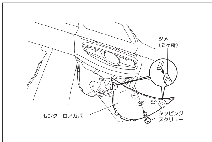
(1) センターロアカバーを取外します。
