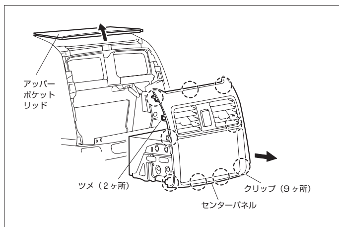
(3) センターパネルA'ssyを取外します。
